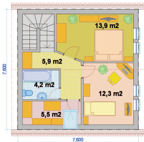
PŮDORYS PODKROVÍ
