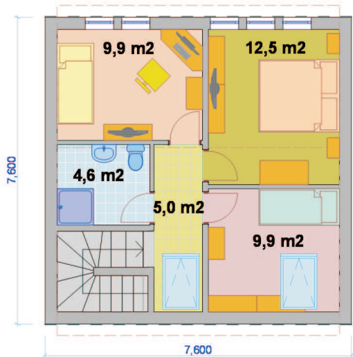
PŮDORYS PODKROVÍ
